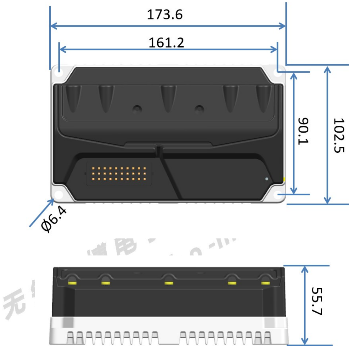
LBMC HK5AE 外形示意图
